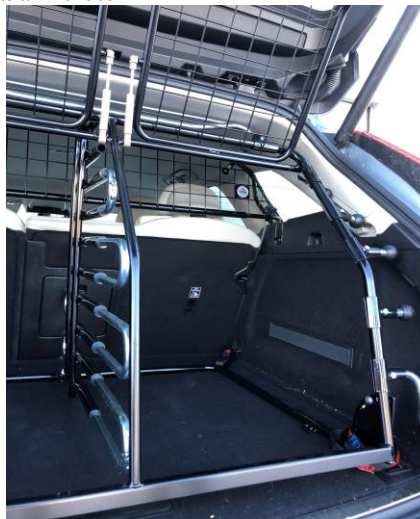
Grind Modell 2 dubbeldörr & avdelare Small i en Volvo XC60 gen II. Bilen är även utrustad med ett modellanpassat skyddsgaller från Artfex. Utfyllnadsrör med knapp utgick 201809 och har ersatts av "Hundben"
